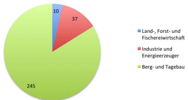
Verbrauch von Grund- und Quellwasser Mio. m 3
