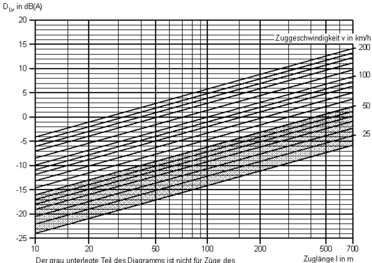
Diagramm II: Korrektur D_{l,v} in dB(A) für unterschiedliche Zuglängen und Zuggeschwindigkeiten
